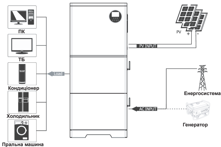
Схема системи
